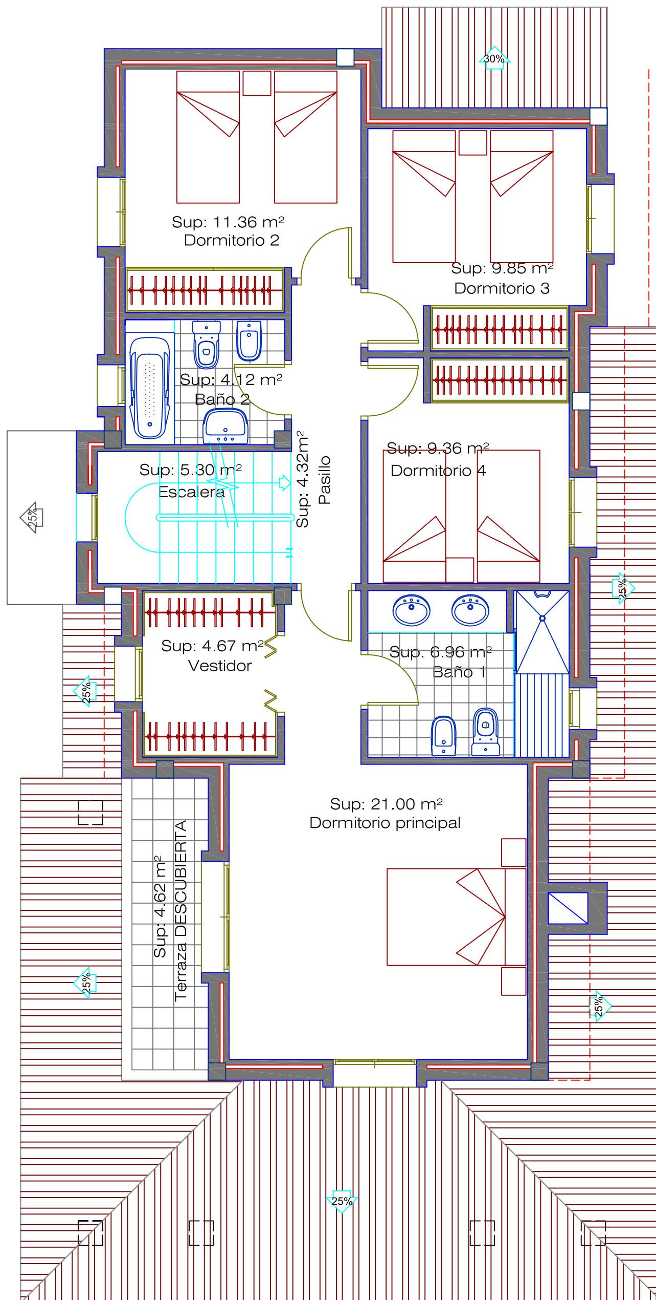
Planta Superior
